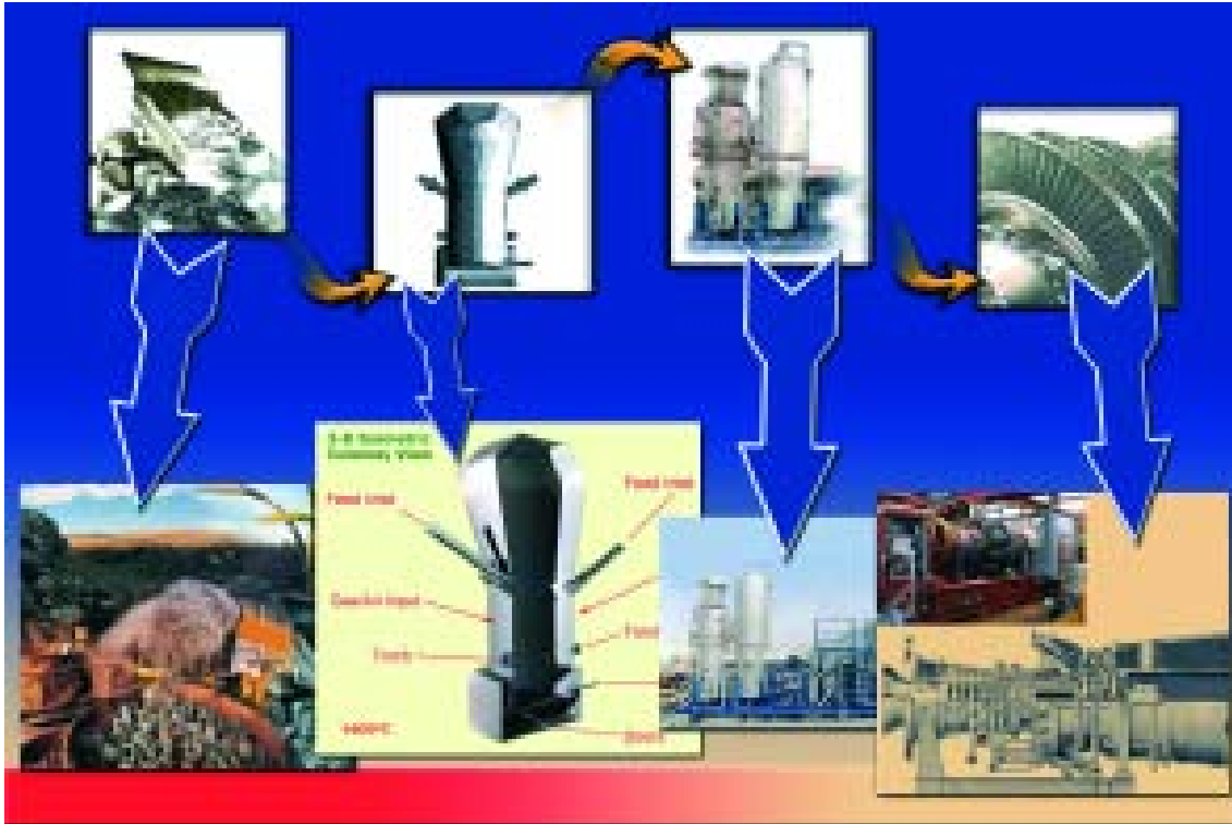
Esquema del proceso de tratamiento de residuos en una planta de gasificación por plasma
